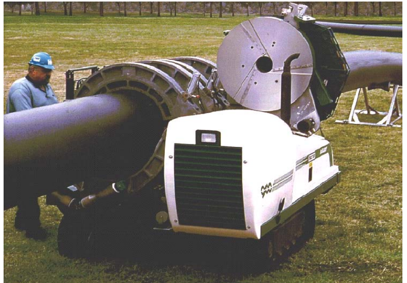
Movimiento hidráulico del espejo y refrentador en
