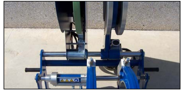
El espejo y refrentador se desplazan por la guía
